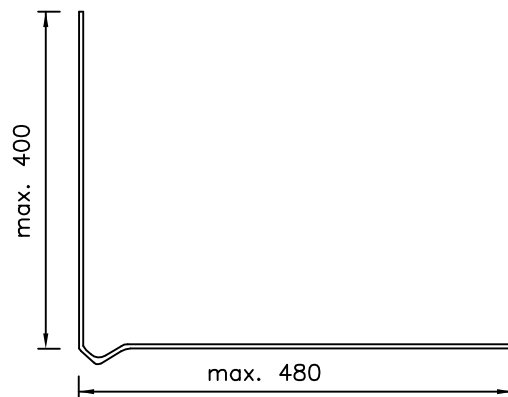
Type Windveerprofiel max. 8,00 meter
