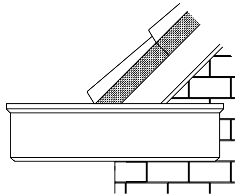
Detail: Type EL 400 met verstekhoek
