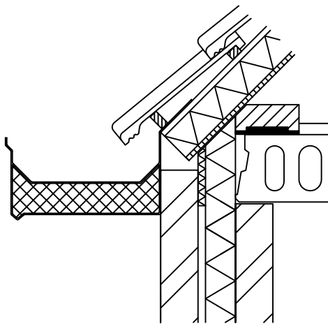
Doorsnede: Type EL 400
